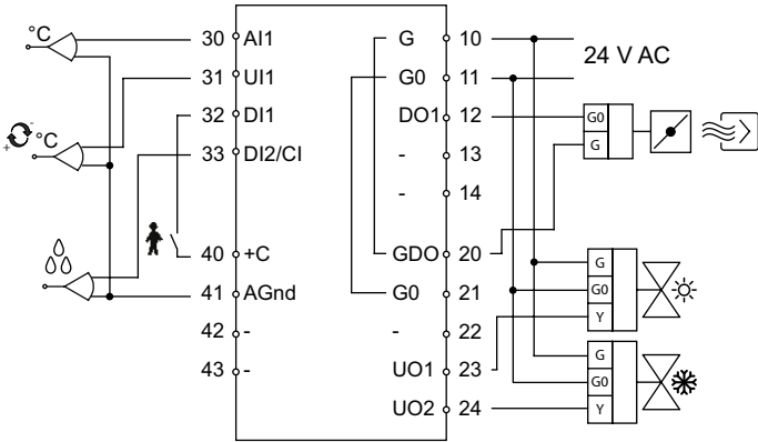
Figure 4. Schéma de connexion de RC-DO
