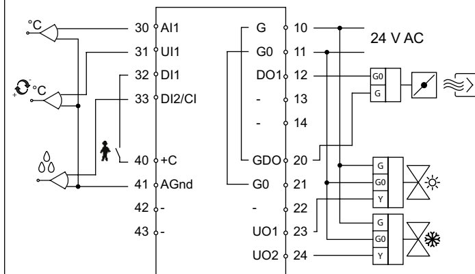
Figur 4. Inkopplingsschema för RC-DO
